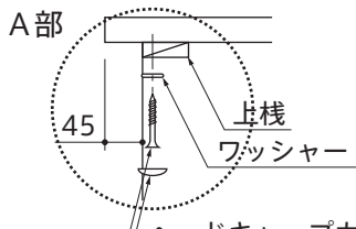
引き出しユニット/ 加熱機器ユニット前面
