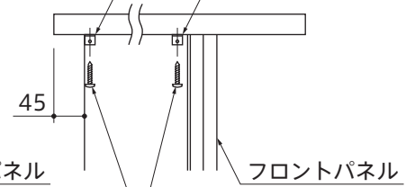
食洗機ユニット前面/後面
