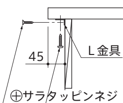
シンクユニット前面
